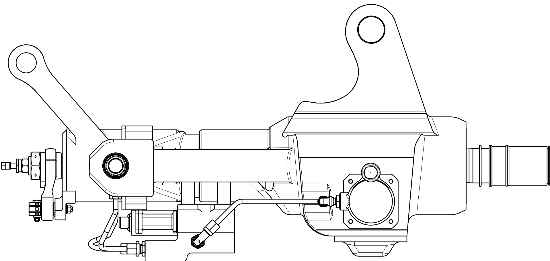
Right view Scale: 1:3
