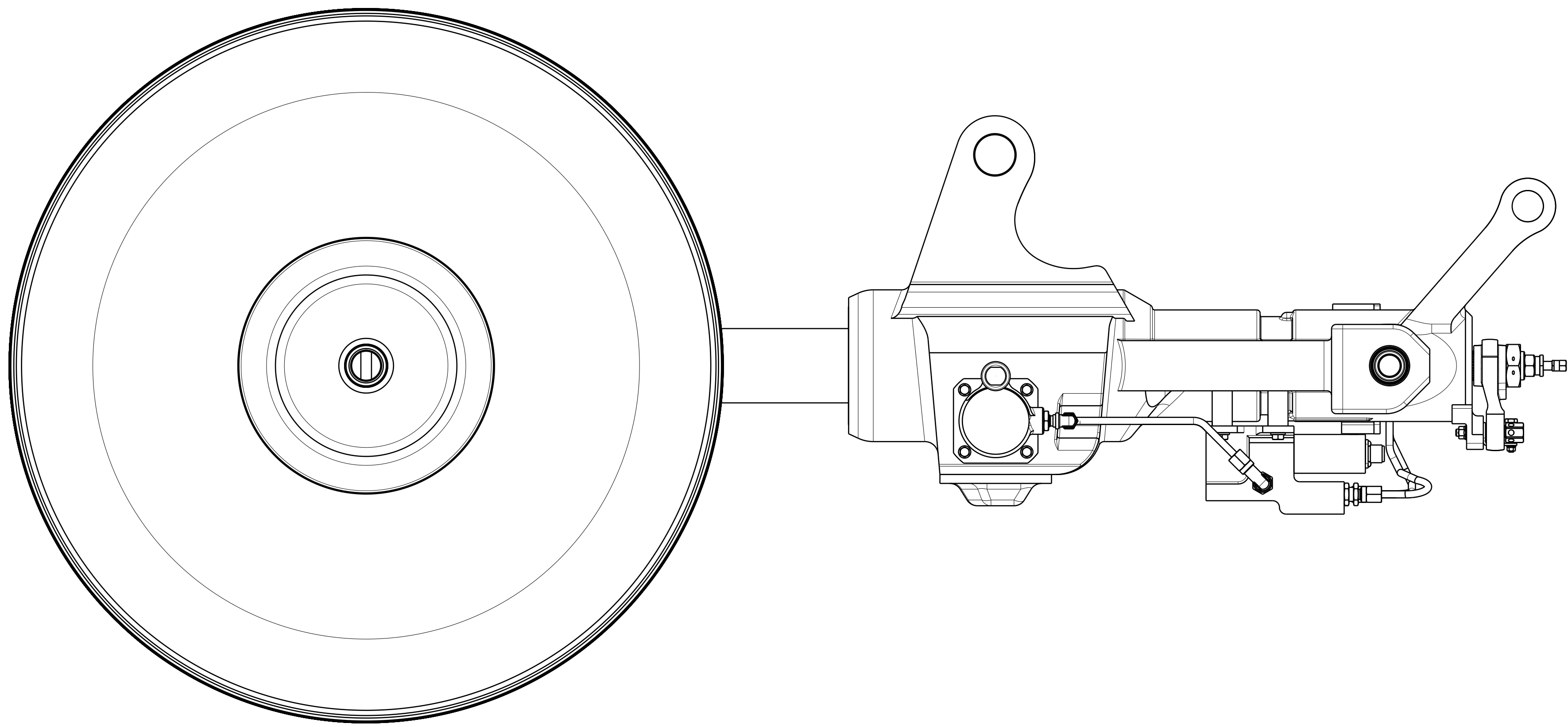
Left view Scale: 1:3
